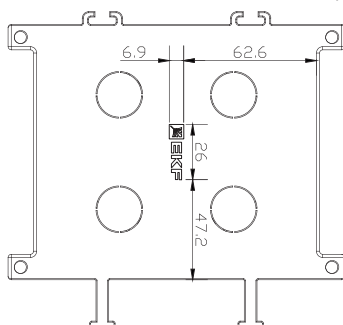
Рис. 15 – Коробка напольная под лючок C-Line WP-6 (арт. cl-knl-6)
