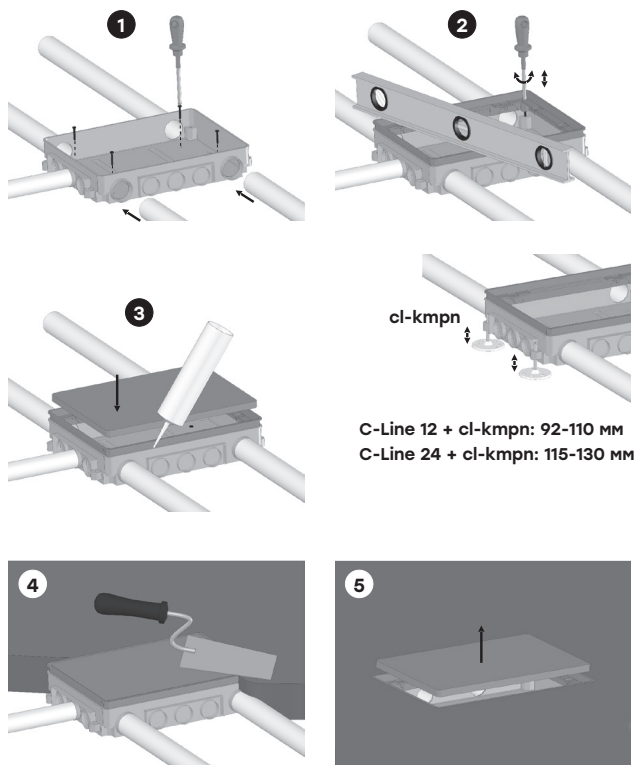
Рис. 16 – Порядок монтажа коробки напольной для лючка в бетонный пол
