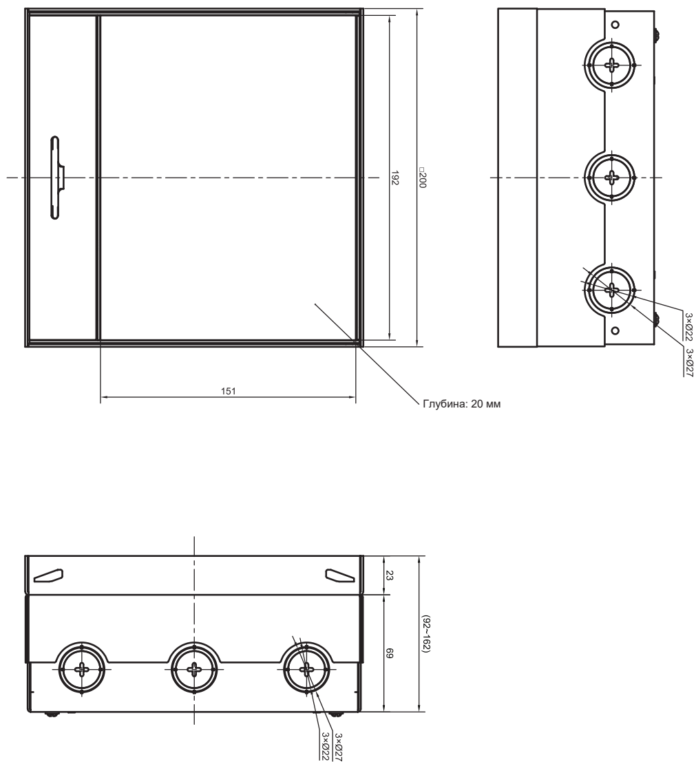
Рис. 13– Лючок металлический C-Line 6 (арт. cl-lnm-6)
