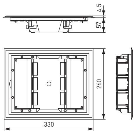
Рис. 1 – Лючок напольный C-Line 12 (арт. cl-ln-12)
