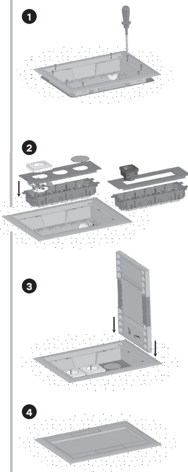
Рис. 17 – Установка лючка
