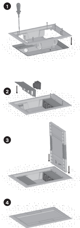
Рис. 17 – Установка лючка
