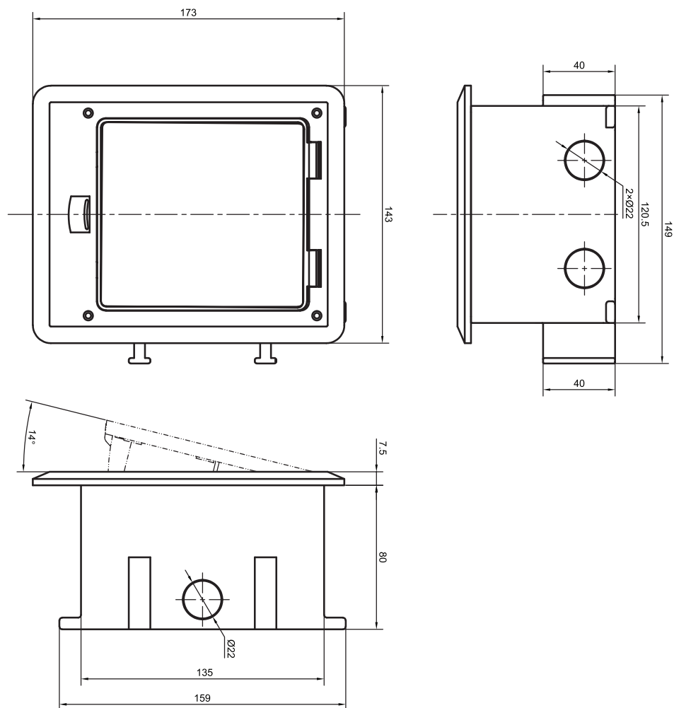
Рис. 14 – Лючок напольный IP66 C-Line WP-6 (арт. cl-lnwp-6)
