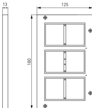
Рис. 12 – Рамка приборная на 12 модулей (арт. cl-рр-12-24)
