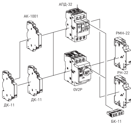
Рис. 1 - Все аксессуары для АПД-32 совместимы с GV2P.
