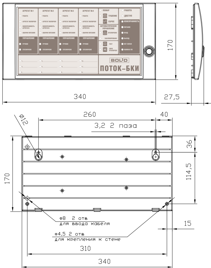
Рисунок 1. Внешний вид, габаритные и установочные размеры блока «Поток-БКИ»
